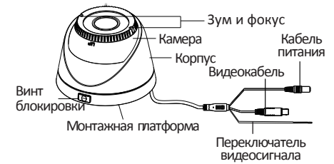
Рисунок 1-2 Камера II типа
