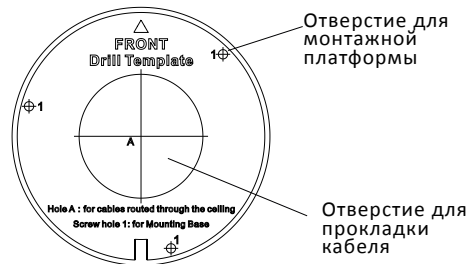
Рисунок 2-5 Шаблон крепления
