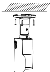
Рисунок 2-2 Установка камеры на потолок
