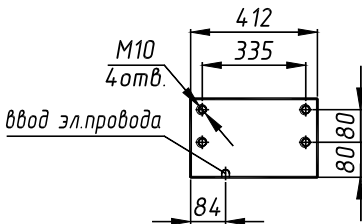
Установочные размеры турникетов "Ростов-Дон Т7М и Т8М"
