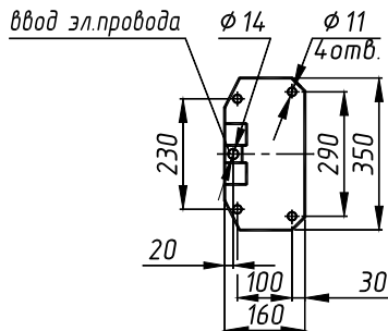
Установочные размеры турникета "Ростов-Дон Т2ММ
