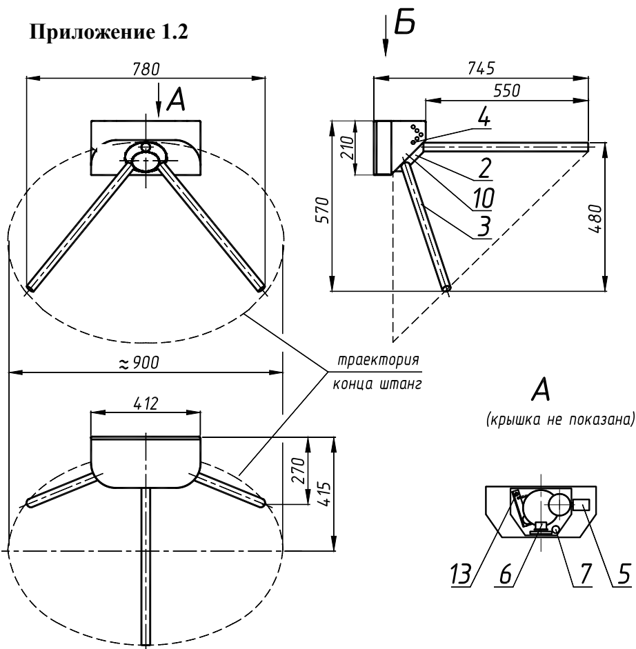
Габаритные размеры турникетов "Ростов-Дон Т7М и Т8М"
