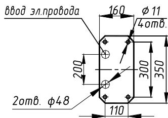
Габаритные размеры турникета "Ростов-Дон Т9М"
