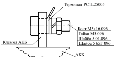
Рисунок 3 – Терминал АКБ
